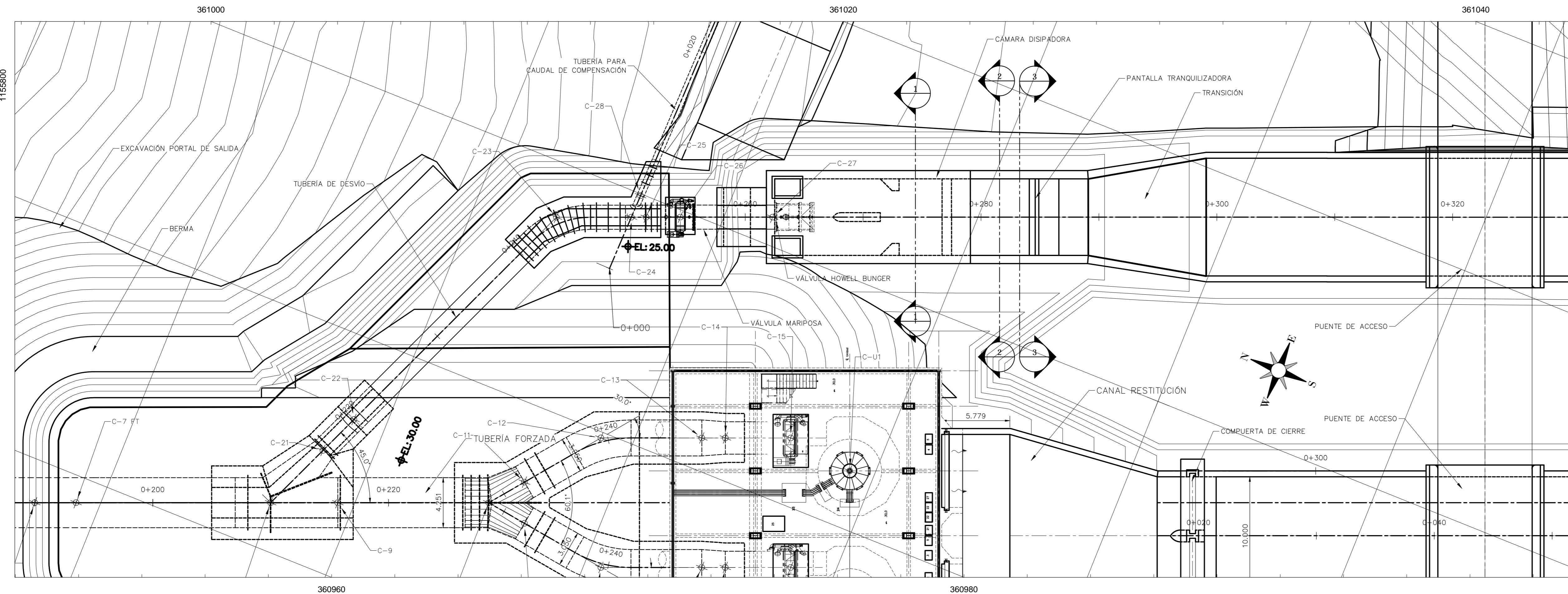
VISTA EN PLANTA DE LA TOMA DE AGUAS, CONDUCCIÓN, DESVÍO, CANAL DE RESTITUCIÓN Y CASA DE MÁQUINAS Escala 1:200
