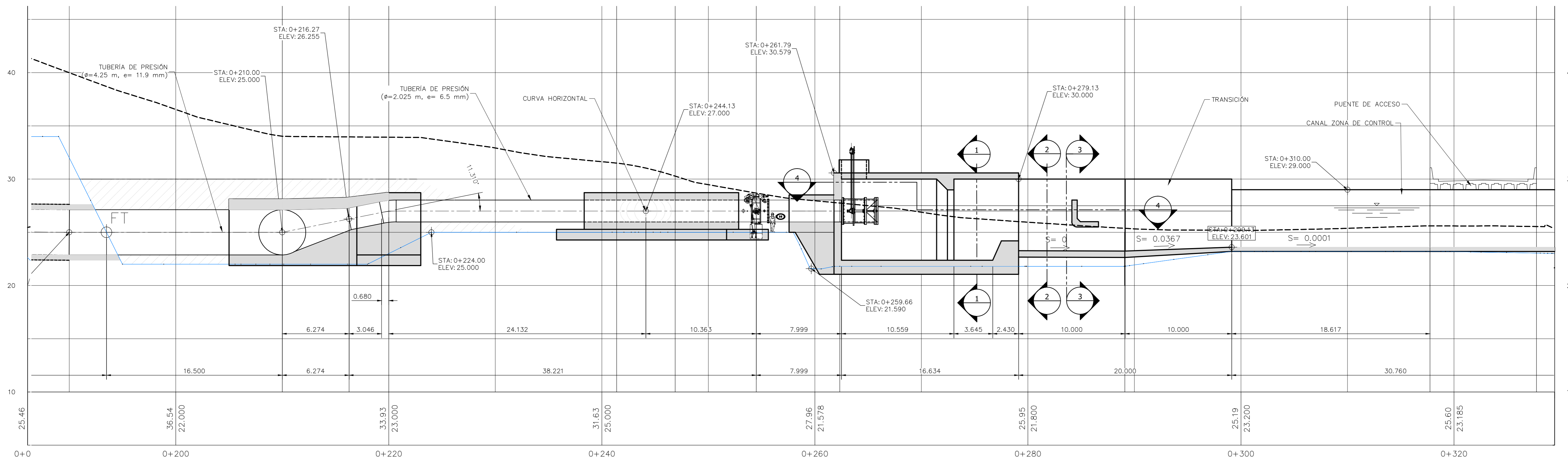
PERFIL LONGITUDINAL DE LA TOMA DE AGUAS, CONDUCCIÓN Y CASA DE MÁQUINAS Escala 1:200
